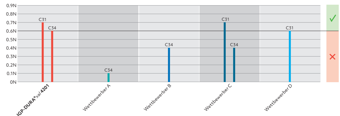
Kratzbeständigkeit «C31/C34 anodisiert»
